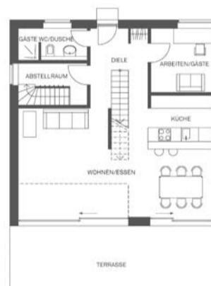
Variohaus EG
